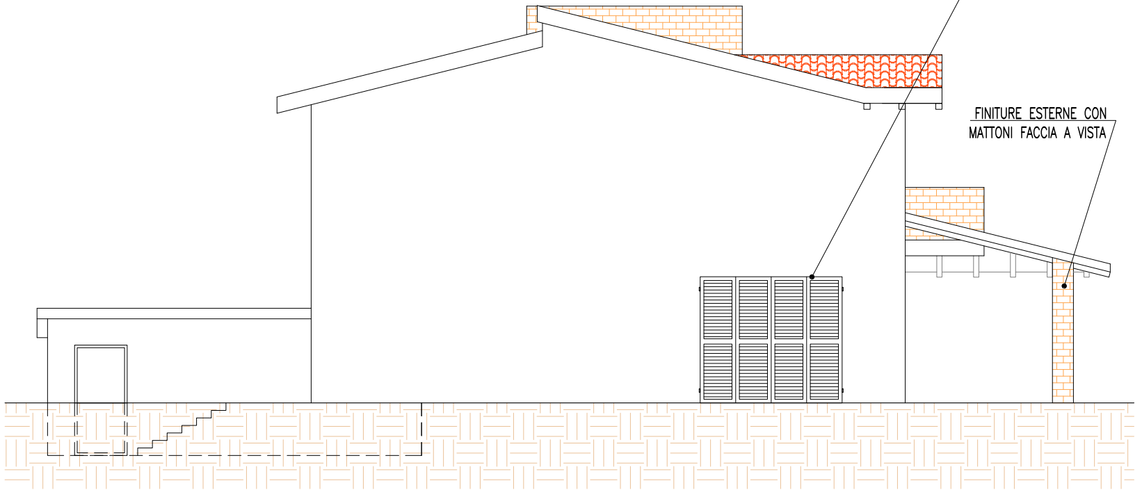
PROSPETTO OVEST
