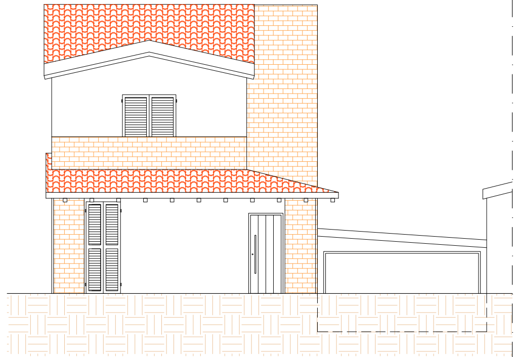
PROSPETTO SUD
