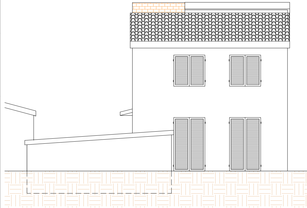
PROSPETTO NORD
