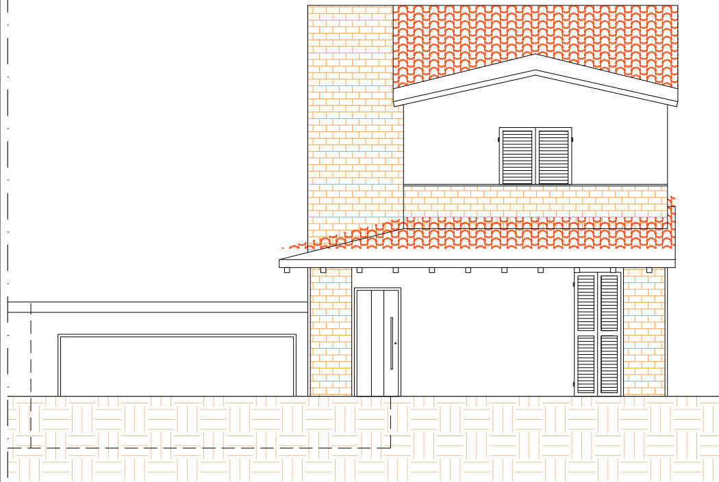
PROSPETTO NORD
