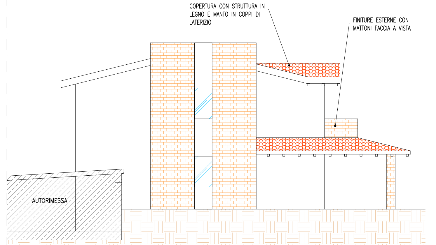
PROSPETTO EST
